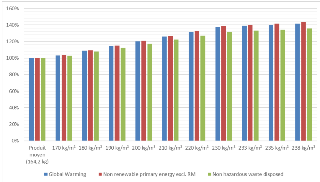
Graphique illustrant la variabilité des résultats d'impacts environnementaux sur 3 indicateurs en fonction de la variation de la masse de briques de terre crue extrudée au mètre carré
