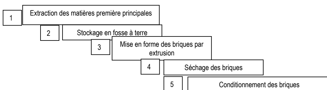
Schéma décrivant le procédé classique de fabrication des briques de terre crue extrudées
